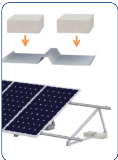
Fijación balastrada
