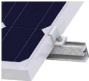
Fijación con grapas superiores
